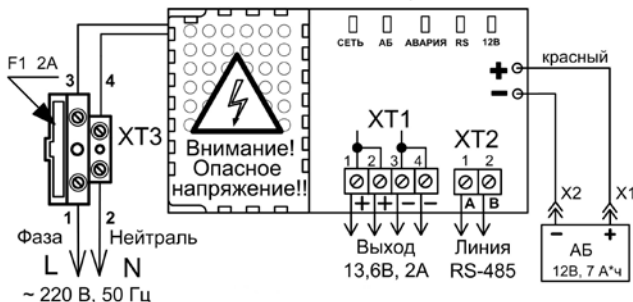
Рисунок 3. Схема подключения «РИП-12 исп.54 (РИП-12-2/7П2-Р-RS)»
